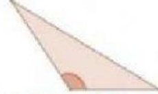
OBTUSÁNGULO
