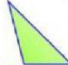
ESCALENO
