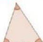
ACUTÁNGULO
