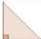
RECTÁNGULO
