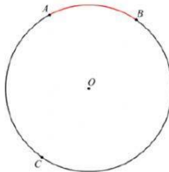
Рис. 4. Дуга окружности
