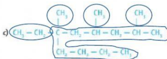
6-etil-2,4,6-trimetildecano
