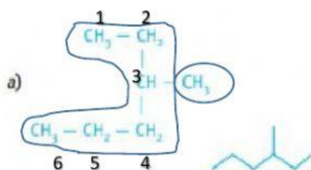
3-metilhexano
