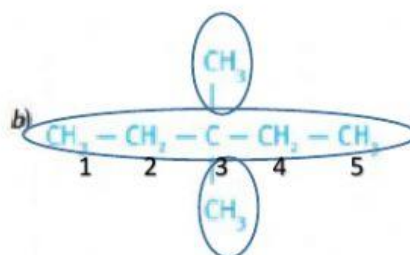
3,3-dimetilpentano
