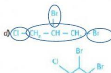
1,2-dibromo-3-cloropropano
