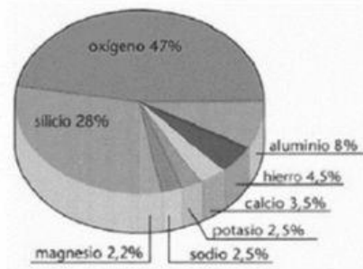
Composición Química de la Corteza Terrestre
