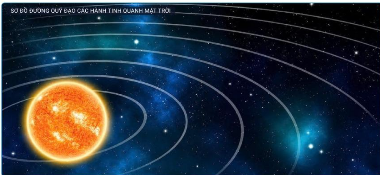
HÌNH ẢNH 8 HÀNH TINH TRONG HỆ MẶT TRỜI (THEO THỨ TỰ)
