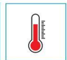
Suhu
