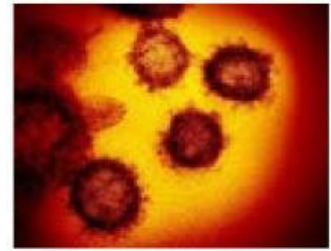
Gambar 2. Mikroskopis Virus corona
