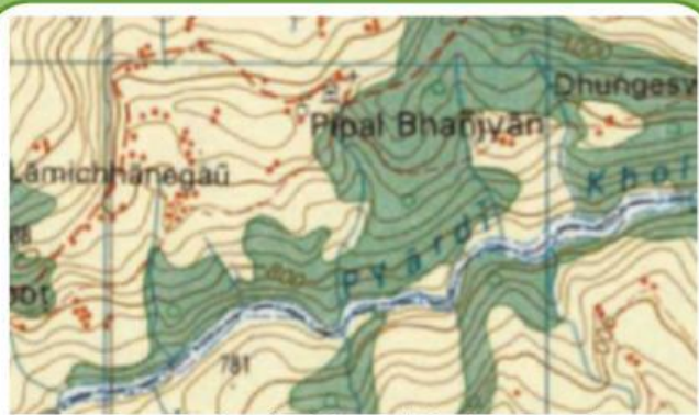
Curvas de Nível de Beshi Shahar, Nepal
