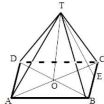
Gambar 4.4. Limas
