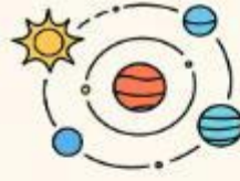
النظام الشمسي
