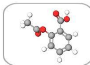
Slika 3: Slika kroglčnega modela molekule acetilsalicilne kisline (povezava do interakt. prikaza)
