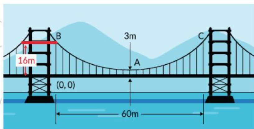
Gambar 6.11 Struktur Jembatan
