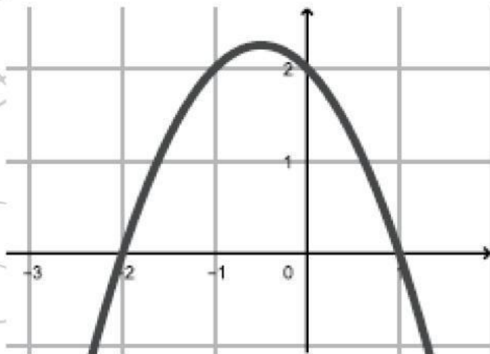
Gambar 6.8 Fungsi Kuadrat dengan c Berbeda
