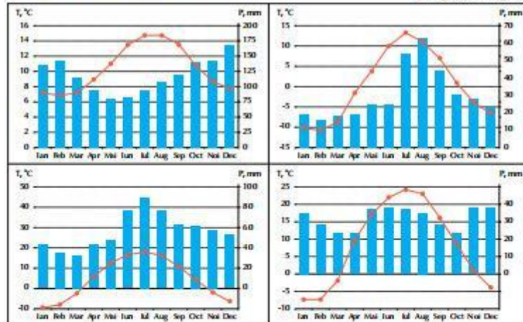
◀ ▼ Fig. 3.66 Climograme
