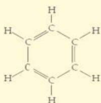
Benzena
