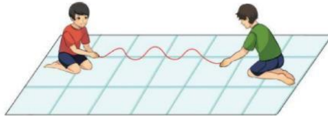
Gambar 10. Membuat gelombang dengan tali Sumber : Buku paket IPA kelas VIII
