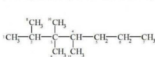
(Senyawa 1)
