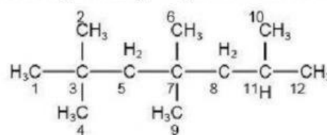
(Senyawa 2)
