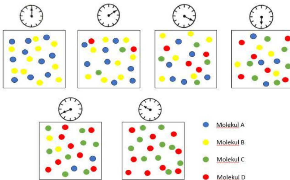
Gambar 2. Perubahan jumlah molekul A + B \rightarrow C + D setiap 10 detik
