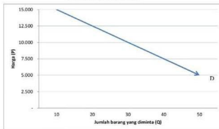
Gambar 2.1 Kurva permintaan
