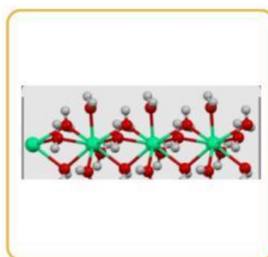
Kalsium Klorida
