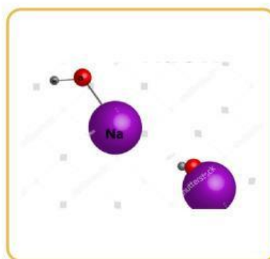
Natrium Hidroksida
