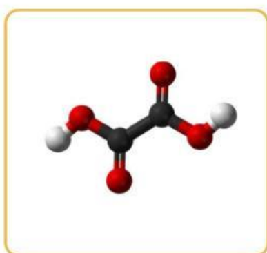
Asam Oksalat
