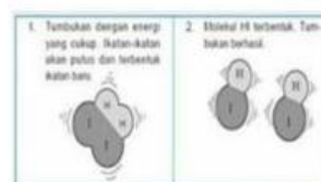
Gambar 2. Tumbukan atom H dan I yang menghasilkan reaksi
