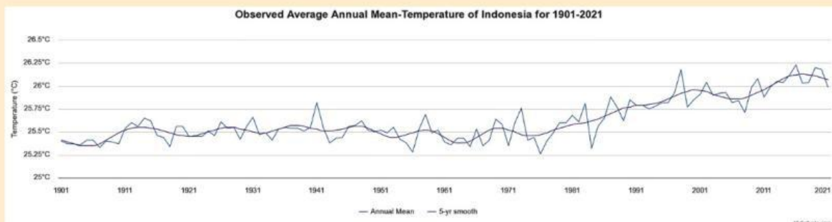
Gambar 1 Rata-rata suhu tahunan Indonesia tahun 1901-2021
