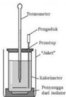
Gambar 9. Kalorimeter Sederhana
