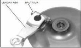
Gambar 5. 16 Pelepasan Plat Indikator
