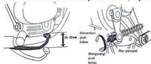
Gambar 5. 15 Penyetel Jarak Main Bebas Pedal
