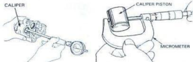
Gambar 5. 10 Pengukuran Kaliper Rem
