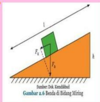
Gambar 3. Benda di bidang miring
