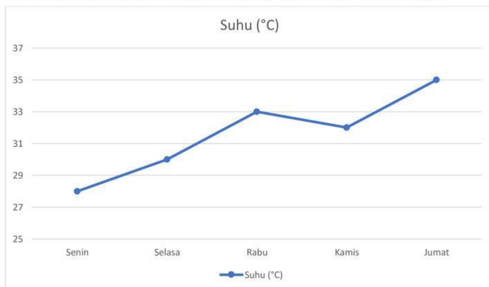
Diagram 2. Kenaikan Suhu Udara
