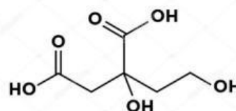
Gambar 7. Struktur molekul asam sitrat Sumber: https://depositphotos.com
