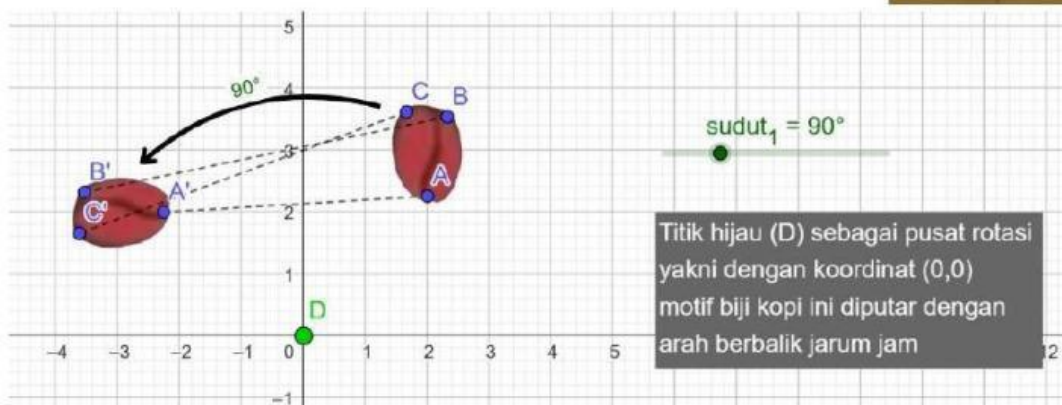
Gambar 2.2. motif batik kopi dirotasi sebesar 90° dengan pusat rotasi di D
