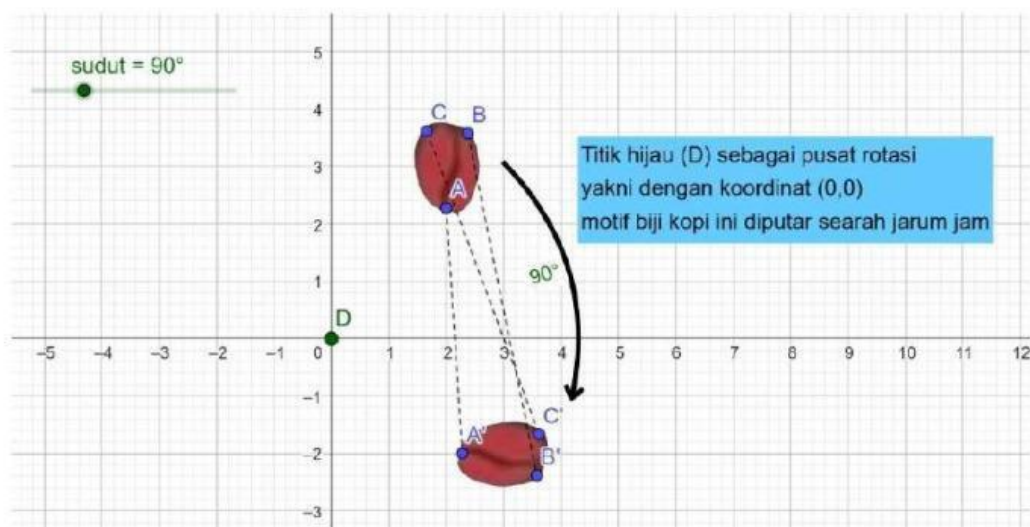
Gambar 2.3. motif batik kopi dirotasi sebesar 90° dengan pusat rotasi di D
