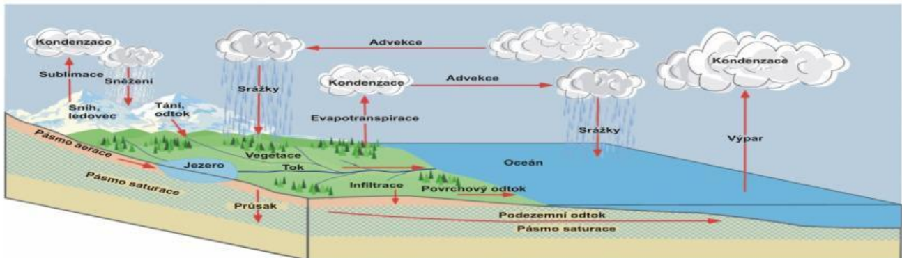
Obr. 10.1 Koloběh vody na zemi
