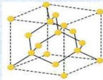
Gambar 6. struktur Intan
