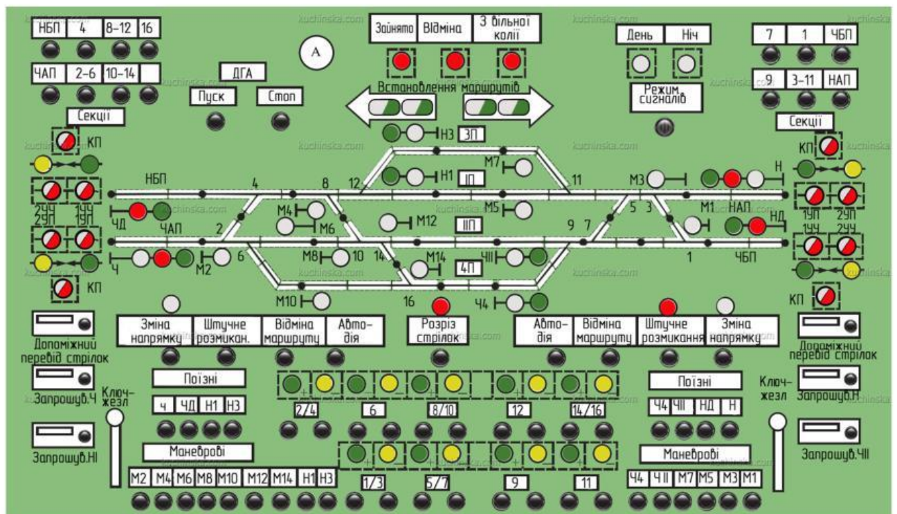
Рис. 10.1 - Пульт-табло жолобкового типу
