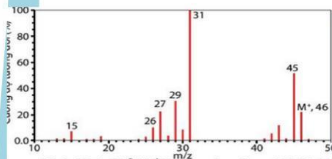
Hình 12.1. Phổ khối lượng của ethanol ( C_2H_6O )
