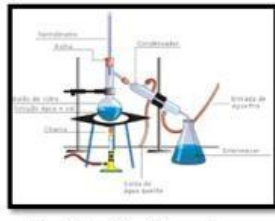
Destilação Simples
