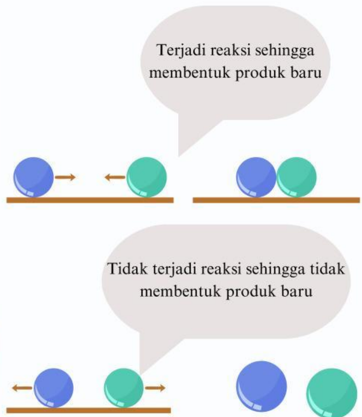
Gambar 2. Tumbukan antar molekul
