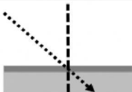
Refracción
