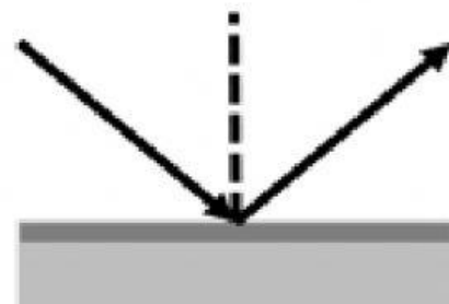
Reflexión
