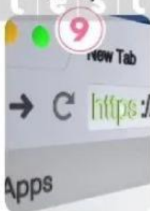
WEB BROWSER
