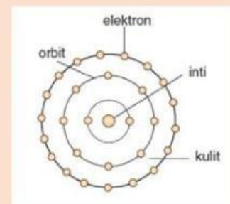
Gambar Atom Bohr
