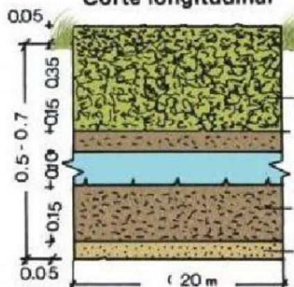
Corte longitudinal
