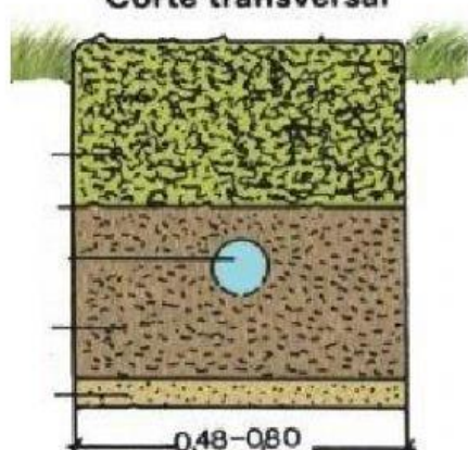
Corte transversal
