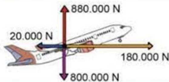
Gambar 3 . Empat gaya pada pesawat terbang
