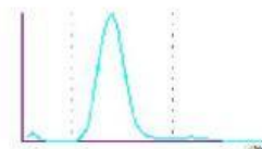
Ιστόγραμμα RBC
