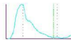
Ιστόγραμμα PLT
