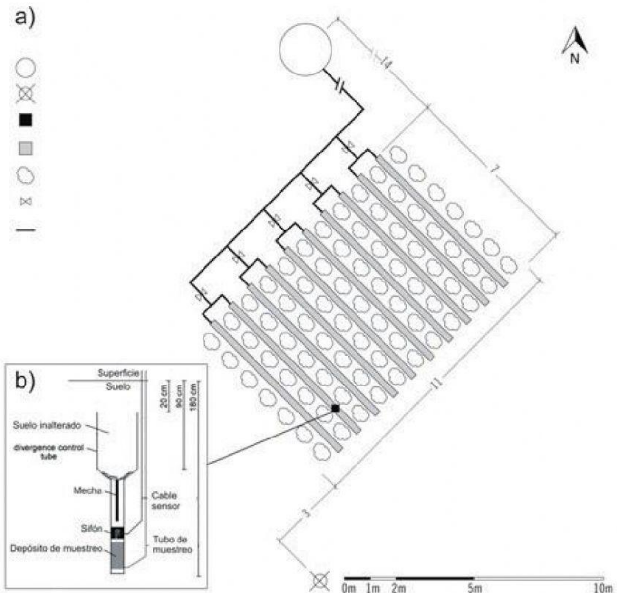
Esquema de un filtro verde por surcos
