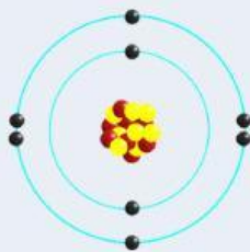
Bohr
