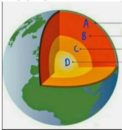
Gambar 1. Lapisan Bumi
