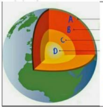
Gambar 1. Lapisan Bumi
