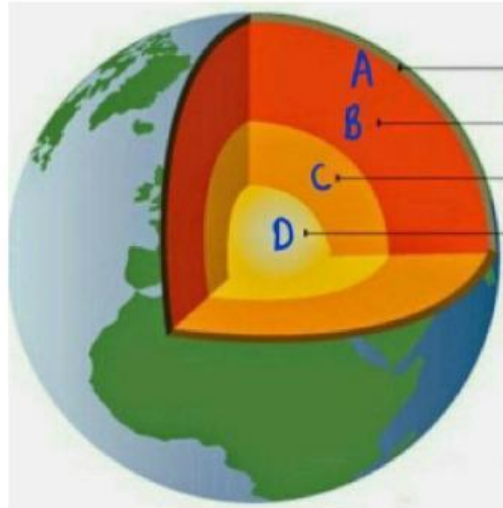
Gambar 3. Lapisan Bumi
