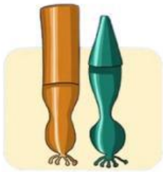
Fotoreseptor (cahaya)
