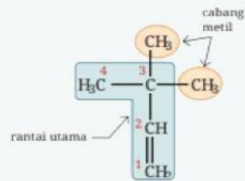
3,3-dimetil-1-butena
