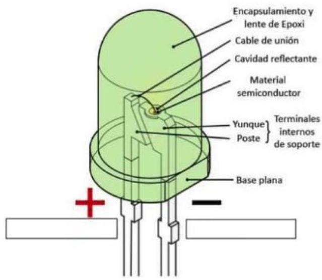
Partes de un Diodo LED
