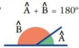
ÁNGULOS SUPLEMENTARIOS
