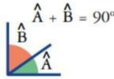
ÁNGULOS COMPLEMENTARIOS
