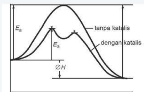
Gambar 6. Pengaruh Katalis terhadap Energi Aktivasi (Sumber : nafiun.com )
