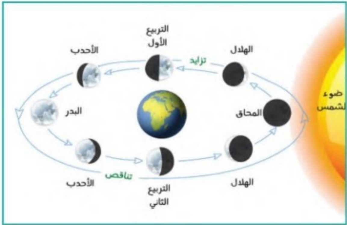
أوجه القمر
