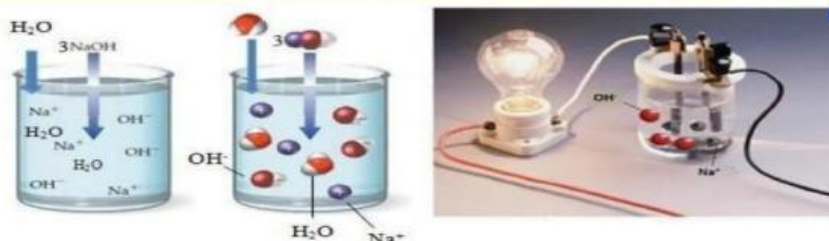
Gambar 24. Ionisasi larutan NaOH dan daya hantar listrik larutan NaOH (Sumber: Nivaldo, 2011)
